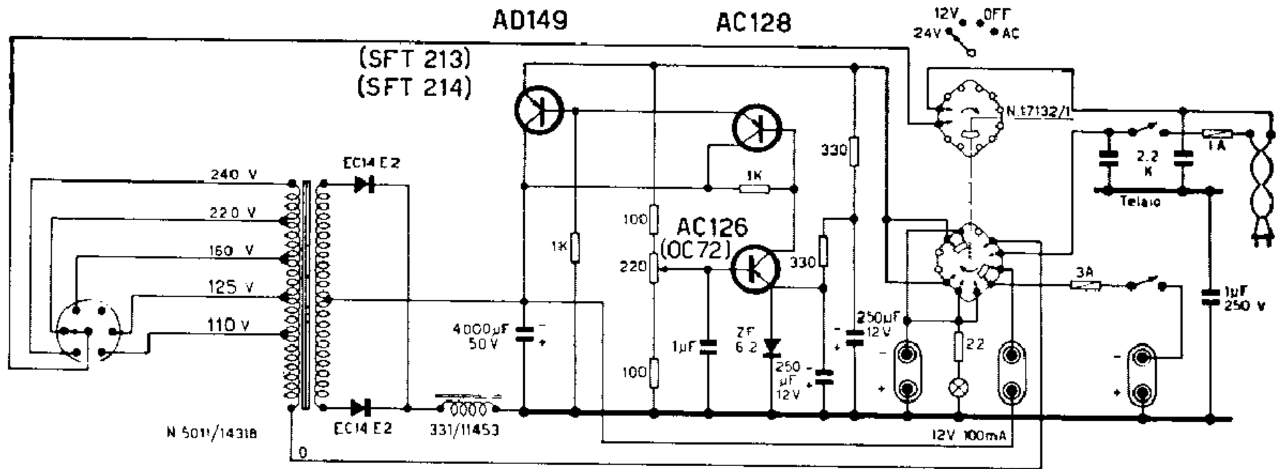
Geloso - Alimentatore mod. G1/121
